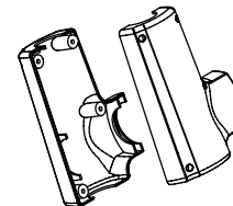
L. Декоративные накладки левого подвижного поручня (2 шт.)
